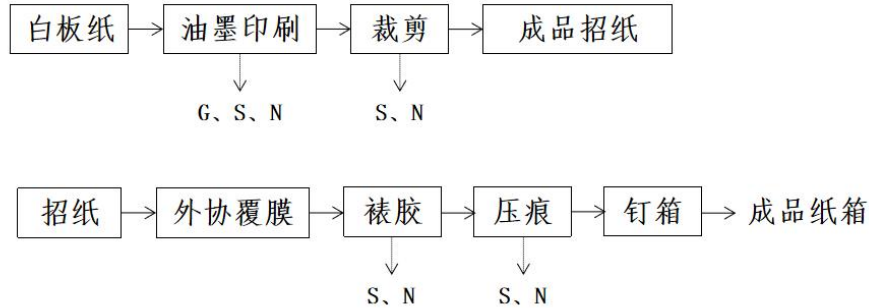
图 1 工艺流程及产污环节图 (G-废气；S-固体废弃物；N-噪声)
